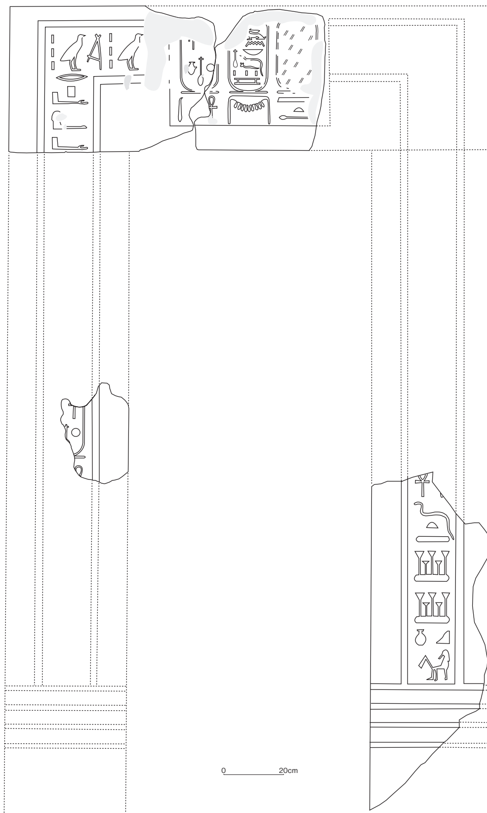
Fig. 12. Porte dans l'enceinte de la chapelle d'Osiris Ounnefer Neb-djeftaou. Schéma de restitution (blocs ON 16, 17, 19 + Cheikh Labib 92CL580), L. Coulon / R. Migalla.
